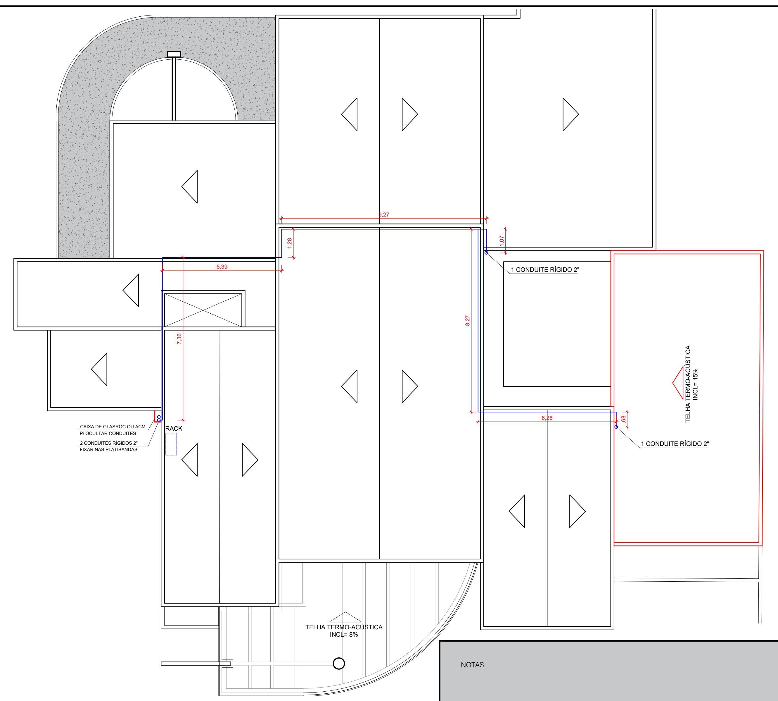
REDE ESTRUTURADA INTERNET ESC. 1:100
