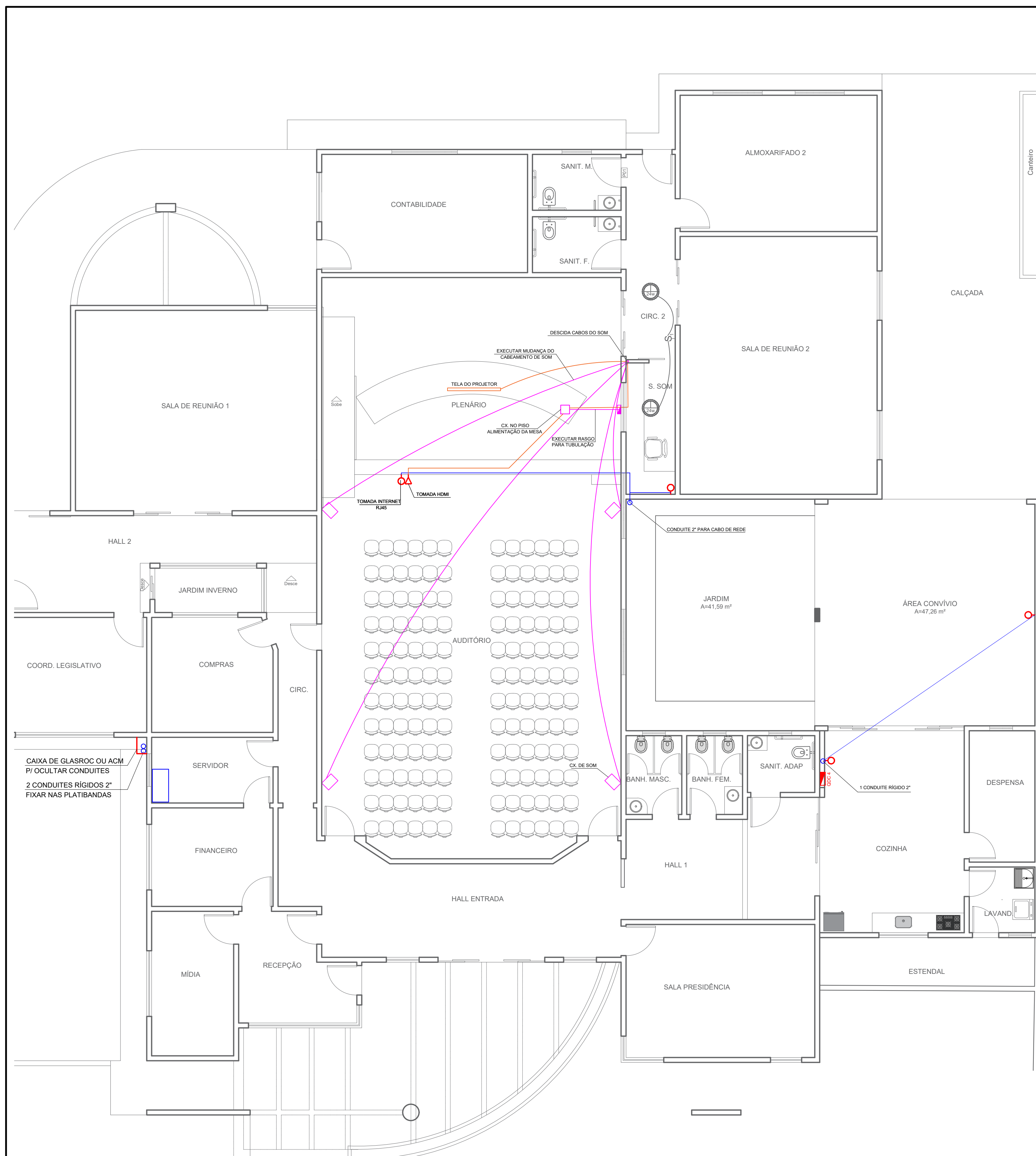
CABEAMENTO INTERNET/SOM/HDMI ESC. 1:75
