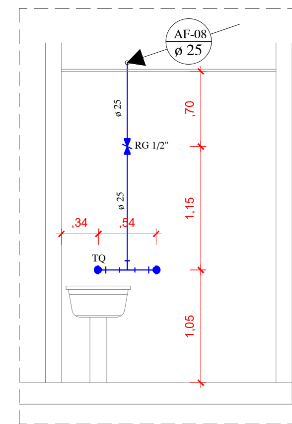
LAVANDERIA VISTA 05 - ESC. 1/35
