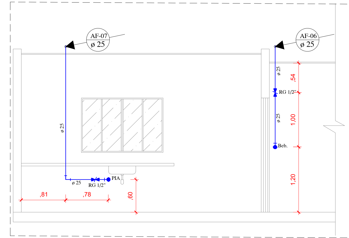
COZINHA VISTA 04 - ESC. 1/35
