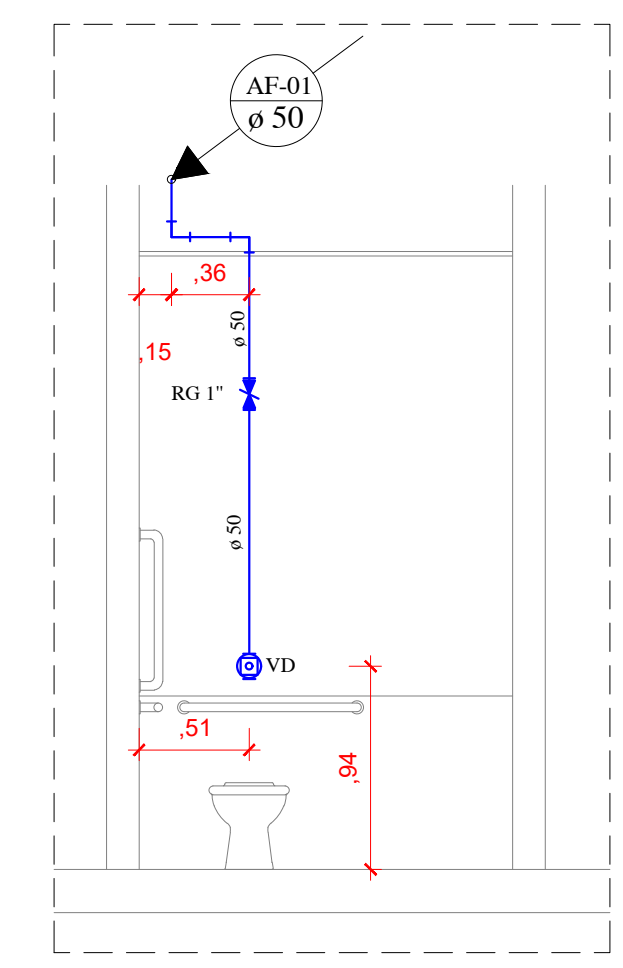
SANT. ADAPT VISTA 01 - ESC. 1/35
