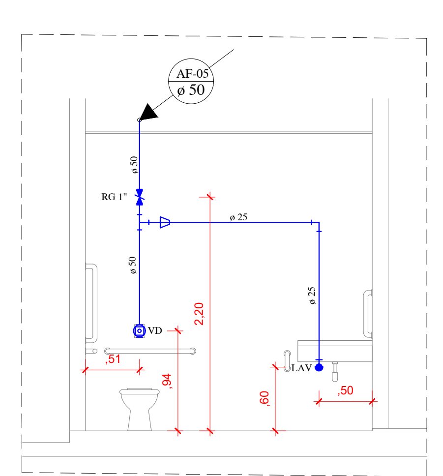
SANT. FEMIN. (SEMELHANTE SANT. MASC.) VISTA 03 - ESC. 1/35
