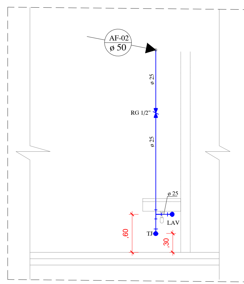
SANT. ADAPT - LADO EXTERNO VISTA 02 - ESC. 1/35
