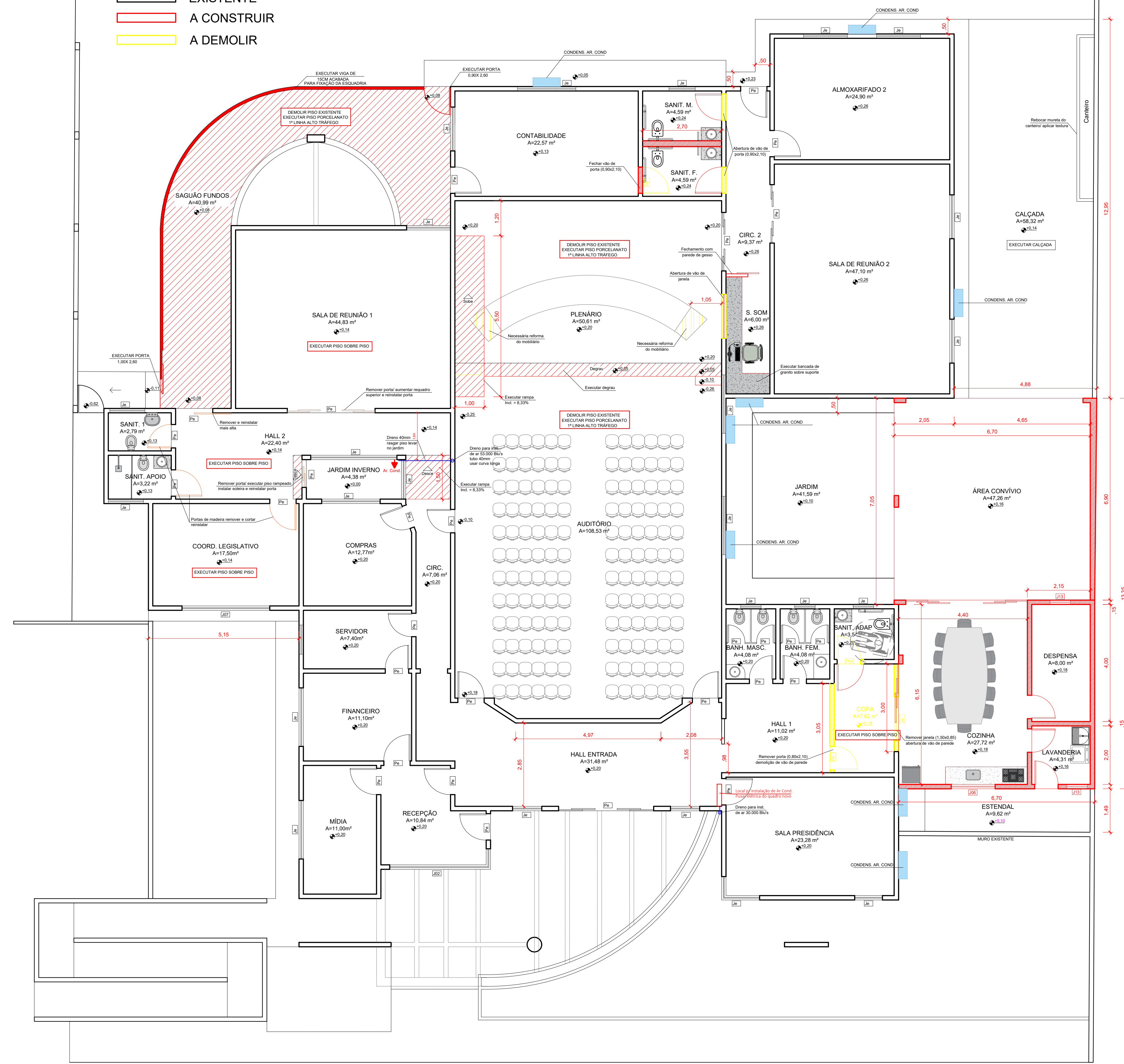
PLANTA CONSTRUÇÃO/DEMOLIÇÃO ESC. 1:75
